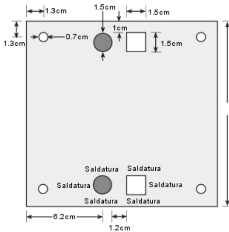
Base del Bersaglio (vista dall'alto)
